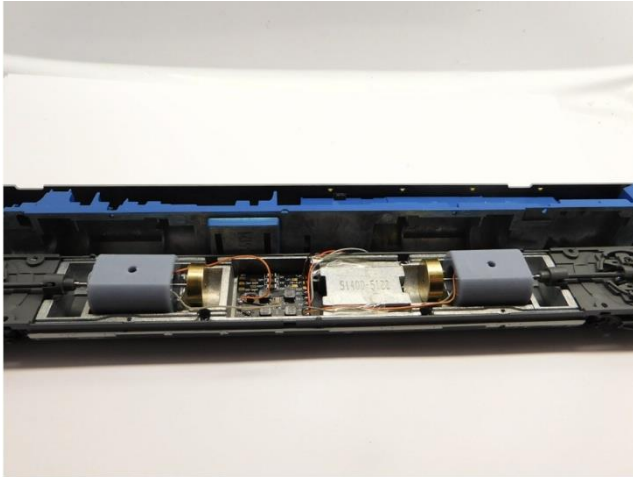
Motor im Motorhalter platzieren Place motors in motor holders Plaats de motoren in de motor houders
