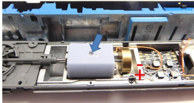
Der Motor wird mit Epoxidkleber oder Sekundenkleber in den Motorhalter eingeklebt The motor is glued into the motor holder with epoxy glue or super glue De motor wordt verlijmd met secondelijm of epoxy lijm
