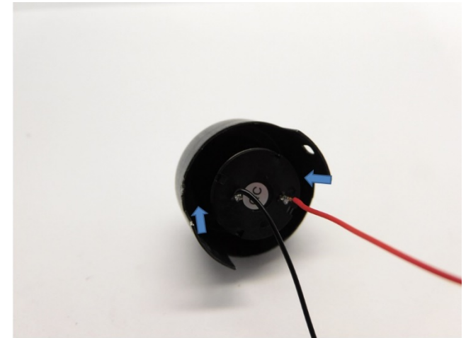
Kleben mit Loctite oder Metal Epoxy Kleber Glue with Loctite or metal epoxy glue Verlijm het met Loctite of epoxylijm voor metaal
