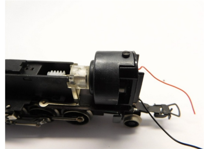
Drehgestell platzieren Mount bogie Plaats het draaitstel
