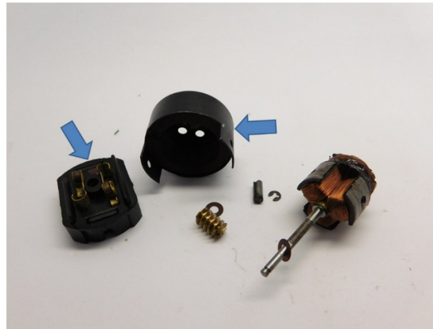
Sie brauchen die Teile wieder You need the parts again Je hebt de onderdelen wederom nodig
