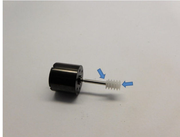
Der Schnecke wird mit Sekundenkleber geklebt The worm gear is glued with super glue Het wormwiel wordt met secondelijm verlijmd
