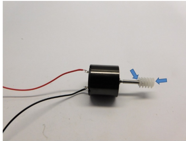
Der Schnecke wird mit Sekundenkleber geklebt The worm gear is glued with super glue Het wormwiel wordt met secondelijm verlijmd
