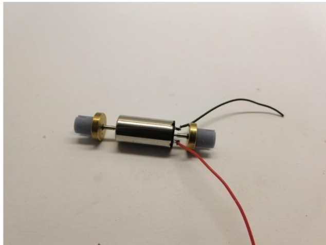
Kleben Sie die Kardankupplungen Glue the cardan couplings Verlijm de cardan koppelingen
