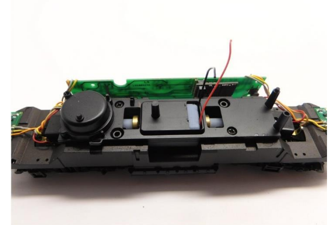
Rahmen platzieren Place the frame Plaats het frame
