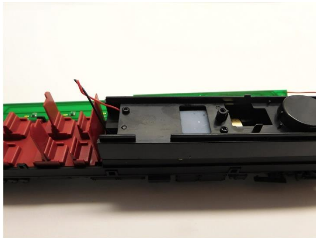
Rahmen platzieren Place the frame Plaats het frame
