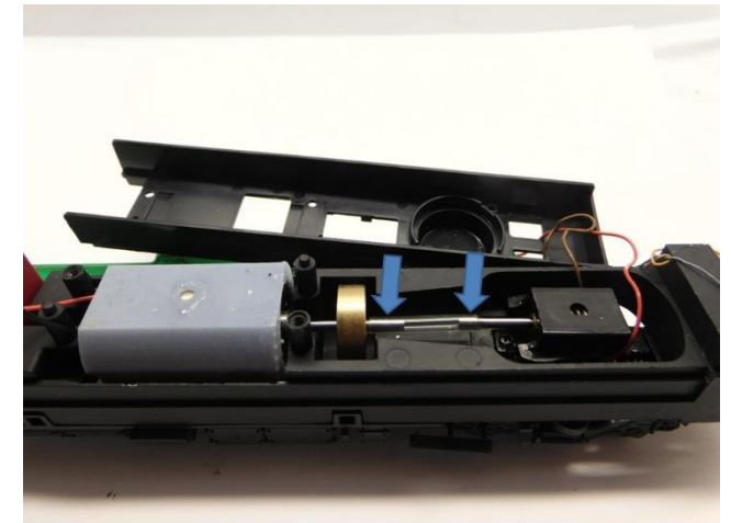
Schlauchkupplung kleben Glue hose coupling Verlijm de slangkoppeling
