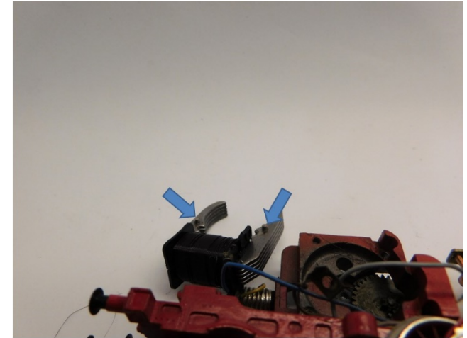
Mit einer Trennscheibe entfernen Remove with cutting disc Verwijder met een slijpschijf
