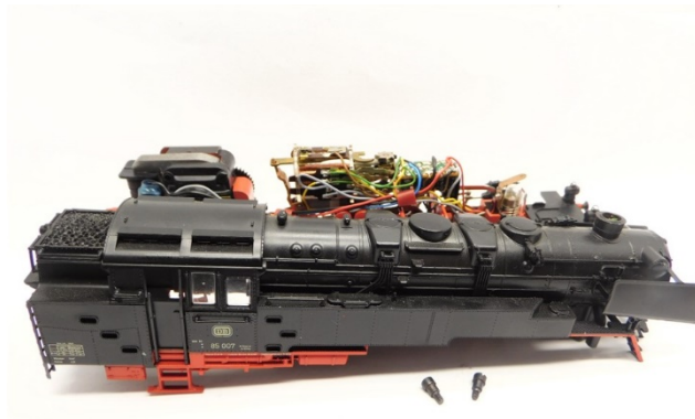
Gehäuse entfernen Remove housing Verwijder de kap
