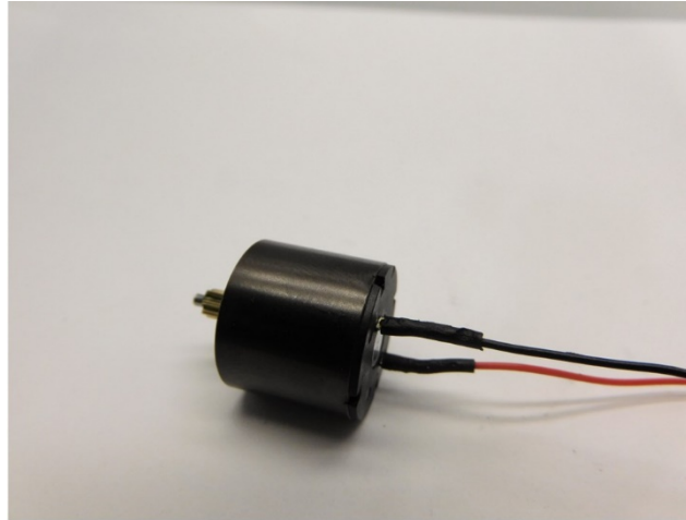
Schrumpfschlauch platzieren Mount shrink tubing Plaats de krimpkousen
