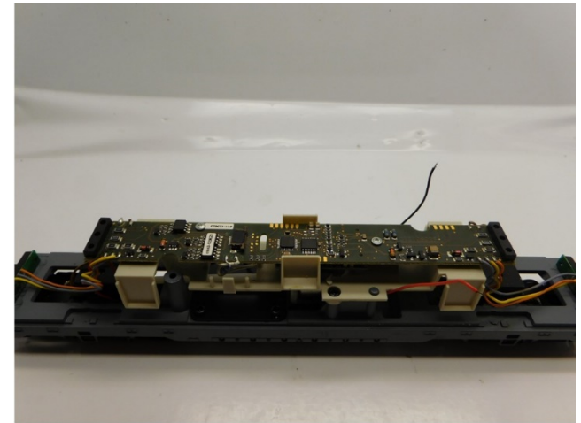
Motor und Platine platzieren Mount the motor and PCB Plaats de motor en de printplaat
