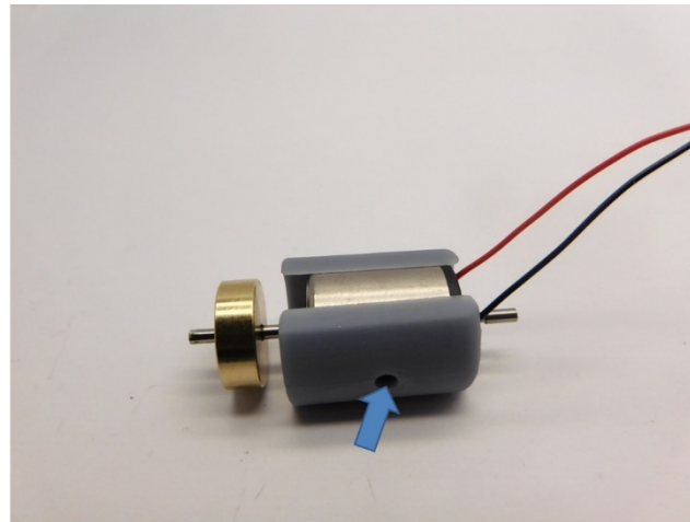
Der Motor wird mit Epoxidkleber oder Sekundenkleber in den Motorhalterteile eingeklebt The motor is glued into the motor holder parts with epoxy glue or super glue De motor wordt in de motorhouderdelen verlijmd met secondelijm of epoxy lijm
