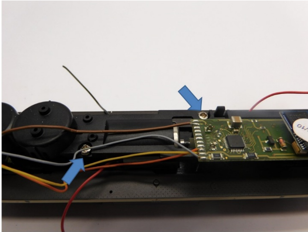
Platzieren Sie die Motorhalterung Mount the motor bracket Plaats de motorhouder
