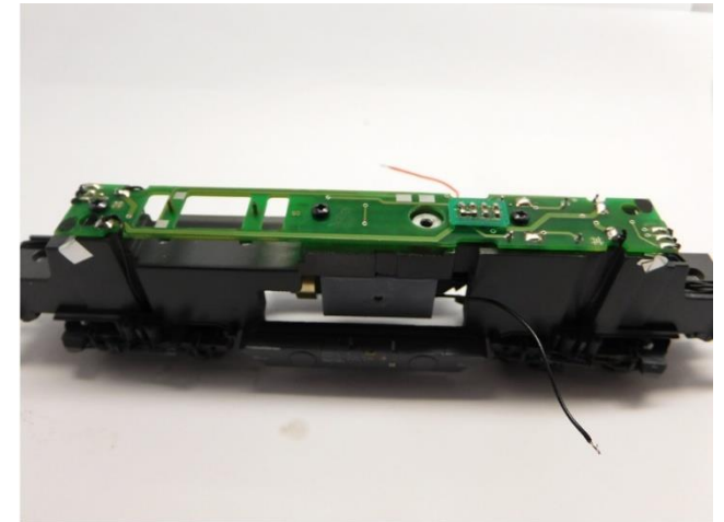
Dreigestell platzieren Mount bogie Plaats het draaistel
