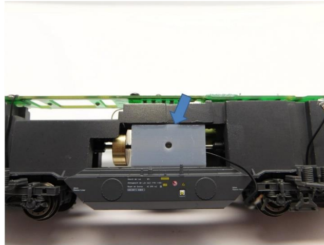
Der Motor wird mit Epoxidkleber oder Sekundenkleber geklebt The motor is glued with epoxy glue or super glue De motor is verlijmd met epoxylijm of secondelijm
