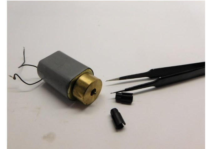
Sie brauchen die Teile wieder. Diese werden mit einer Pinzette entfernt You need the parts again. They can be removed with tweezers Je hebt deze onderdelen wederom nodig. Ze worden met een pincet verwijderd
