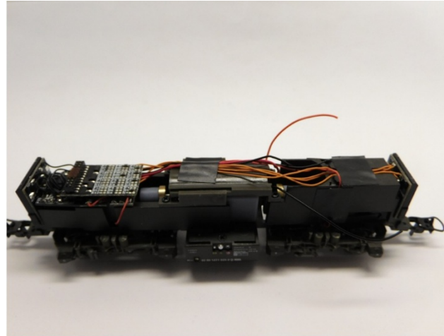
Motorklemme platzieren Place the motor clamp Plaats de motor klem
