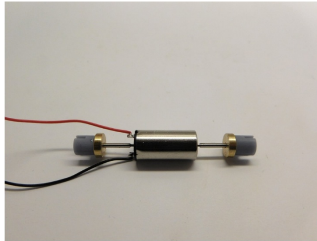
Kardankupplungshalter kleben Glue cardan coupler pockets Verlijm de kardan koppelingshouders
