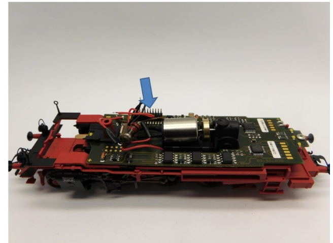
Hinter den Motor passt nur ein kleiner PLUX22-Decoder! Only a small PLUX22 decoder fits behind the motor! Achter de motor past alleen een kleine PLUX22 decoder!
