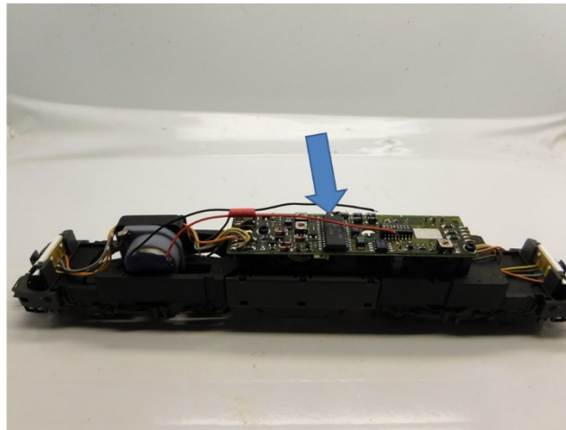
Die alte C-Sinus Leiterplatte muss durch ein Decoder ersetzt werden! The old C-Sinus PCB must be replaced by a decoder! De oude C-Sinus printplaat moet vervangen worden door een decoder!
