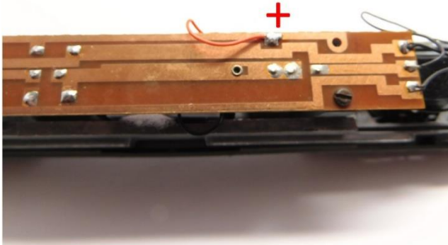
Drähte löten Solder the wires Soldeer de draden
