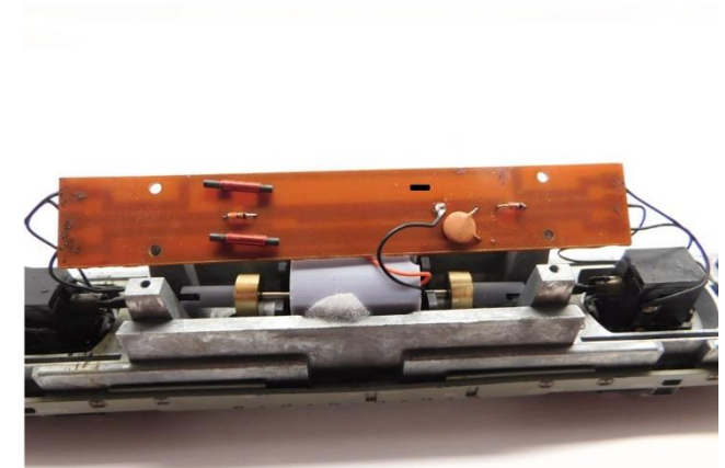
Drähte löten Solder the wires Soldeer de draden
