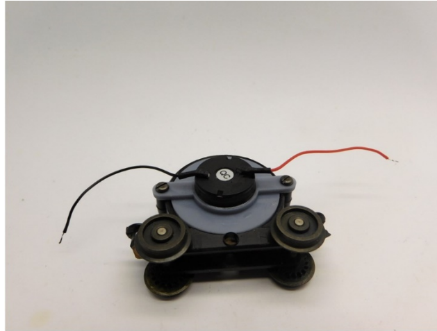
Drähte biegen Bend the wires Buig de draden
