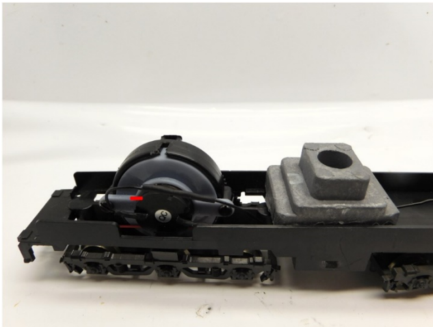
Motor platzieren Mount the motor Plaats de moto
