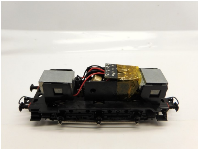
Platzieren Sie die Platine und den Gewicht Mount the PCB and the weight Plaats de printplaat en het gewicht
