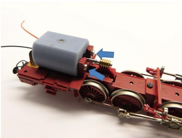
Motorplatte platzieren Mount the motor plate Plaats de motor
