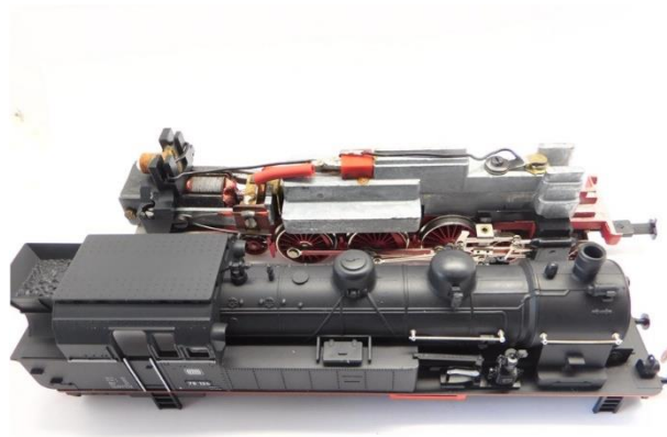
Gehäuse entfernen Remove housing Verwijder de kap
