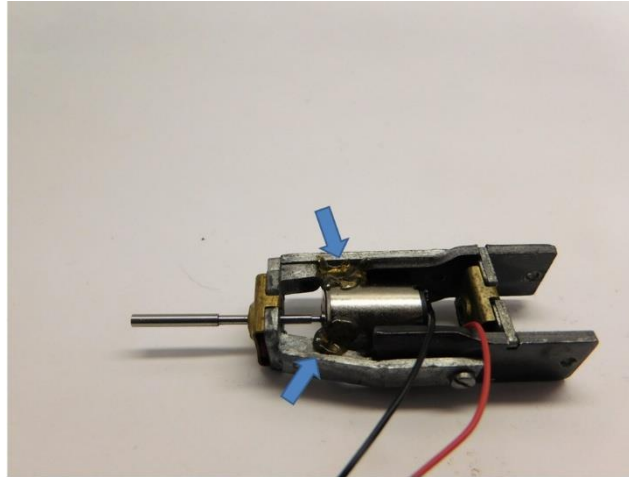
Motor kleben mit Heißkleber Glue the motor with hotmelt Lijm de motor
