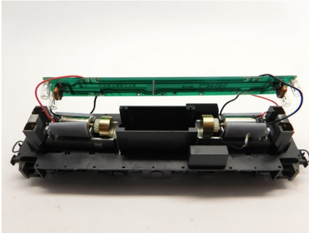
Motoren platzieren Place the motors Plaats de motoren
