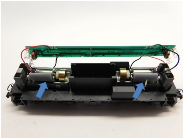
Motoren Kleben Glue the motors Lijm de motor
