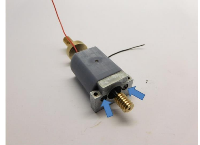
Motorplatte platzieren Mount the motor plate Plaats de motorhouder
