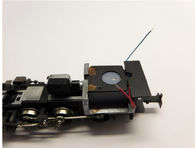
Abdeckplatte platzieren Mount the cover plate Plaats de afdekplaat
