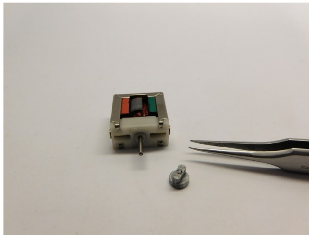
Sie brauchen dieses Teil wieder. Diese wird mit einer Pinzette entfernt You need the part again. It can be removed with tweezers Je hebt dit onderdeel wederom nodig. Het kan met een pincet verwijderd worden
