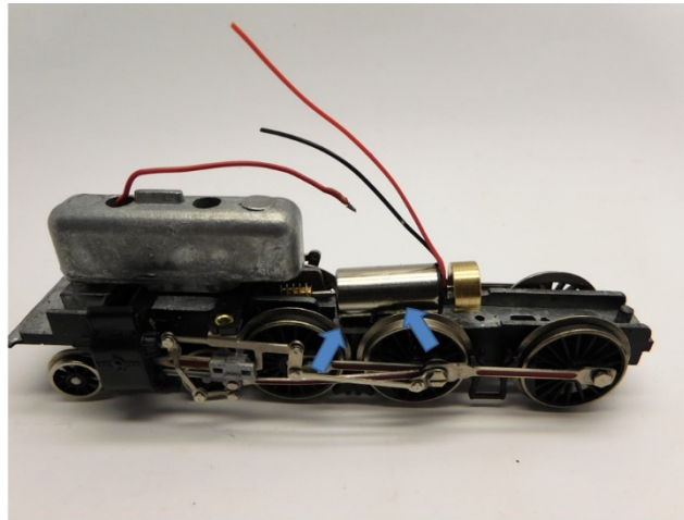
Der Motor wird mit Metallkleber in den Lok eingeklebt The motor is glued into the locomotive with metal glue De motor wordt in de loc met metaallijm verlijmd
