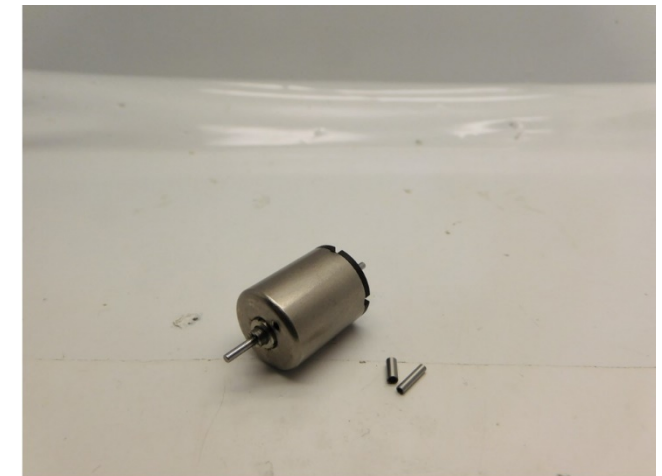
Metal Teile werden mit Loctite oder Metal Epoxy Kleber verklebt Metal parts are glued with Loctite or metal epoxy glue Metalen onderdelen worden gelijmd met metaallijm of epoxylijm voor metalen
