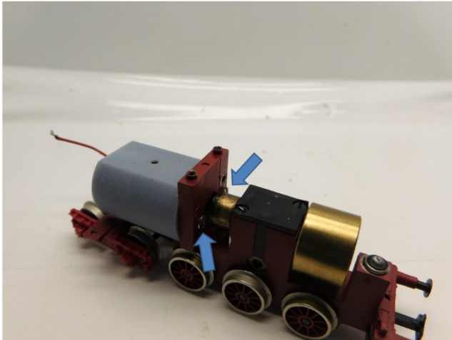
Platzieren Sie den Motorhalter in die Lok Mount the motor holder in the locomotive Plaats de motorhouder in de locomotief
