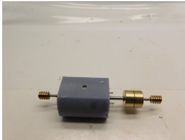
Motor im Motorhalter platzieren Place the motor in motor holder Plaats de motor in de motor houder
