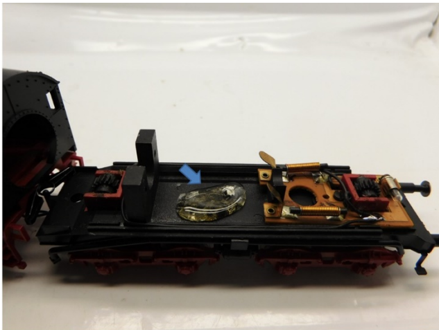
Heißkleber auf den Boden Hot glue on the bottom Smeltlijm op de bodem
