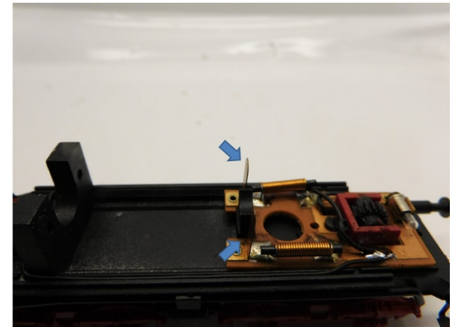
Alter Motorkontakte biegen Bend old motor contacts Buig de oude motor contacten
