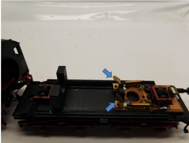
Alter Motorkontakte biegen Bend old motor contacts Buig de oude motor contacten
