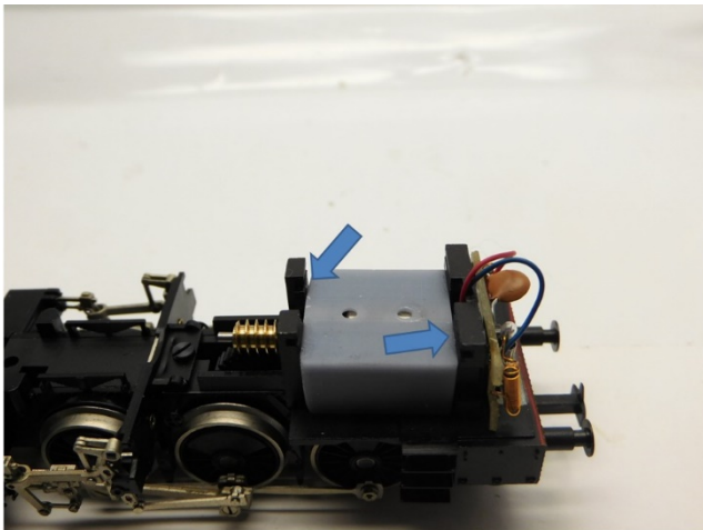
Die Motorhalter kleben Glue the motor holder Verlijm de motor houder
