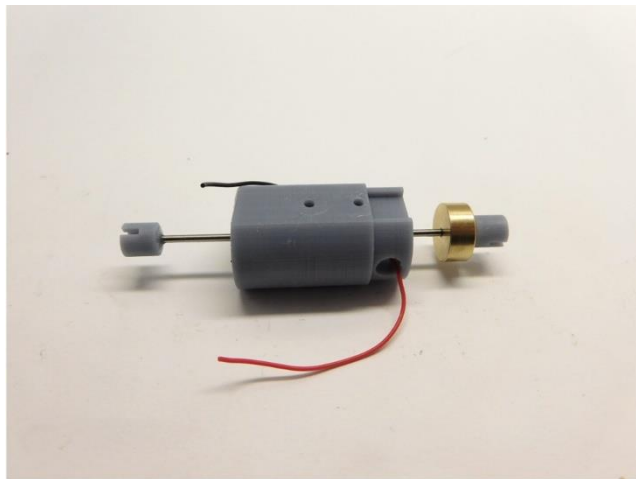
Kardankupplungen kleben Glue the cardan couplers Verlijm de cardan koppelingen
