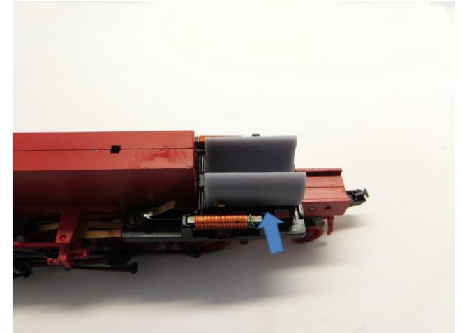
Motorhalter kleben Glue motor holder Verlijm de motor houder
