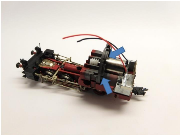
Der Motor wird mit Epoxidkleber oder Sekundenkleber geklebt The motor is glued with epoxy glue or super glue
