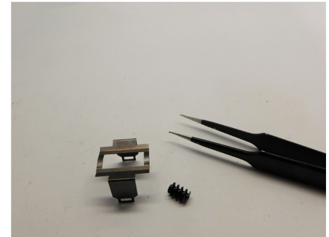
Sie brauchen dieses Teil wieder. Es wird mit einer Pinzette entfernt You need the part again. It can be removed with tweezers Je hebt dit onderdeel wederom nodig. Het kan met een pincet verwijderd worden
