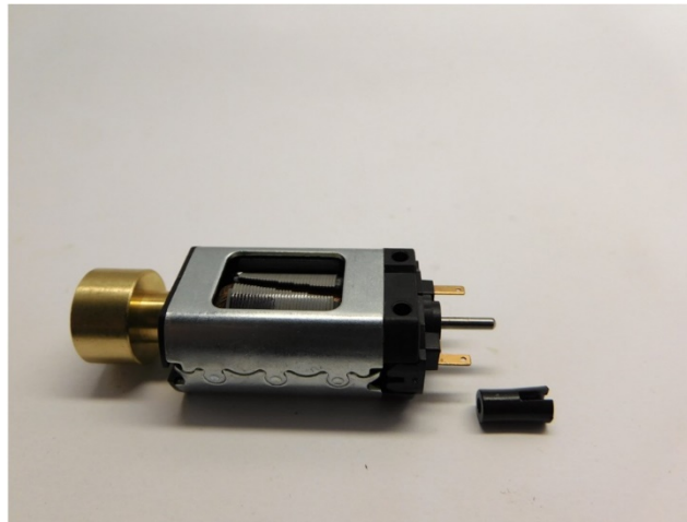
Sie brauchen dieses Teil wieder. Diese wird mit einer Pinzette entfernt You need the part again. It can be removed with tweezers U heeft het onderdeel weer nodig. Het wordt met een pincet verwijderd
