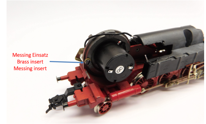
Drähte löten Solder the wires Soldeer de draden
