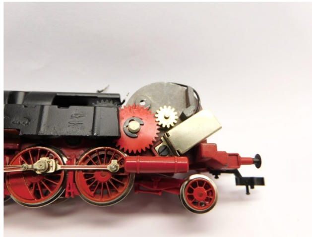
Platzieren Sie das Ritzel Mount the gear Plaats het tandwiel
