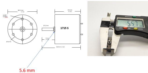
Maße prüfen Check dimensions Controleer de maatvoering
