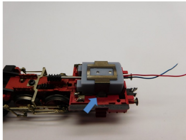
Platzieren Sie den Motorklemme Mount the motor clamp Plaats de motor klem
