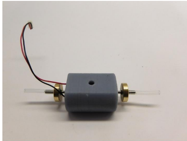
Schlauchkupplungen platzieren Mount hose couplings Monteer de slangkoppelingen
