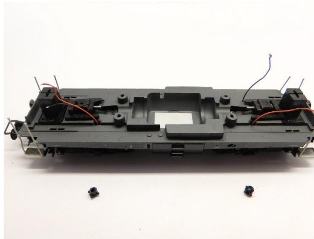
Ausbau Kardankupplungen Take out cardan couplers Verwijder de cardan koppelingen
