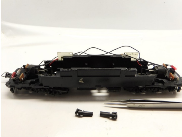
Ausbau Kardankupplungen Take out cardan couplers Verwijder de cardankoppelingen
