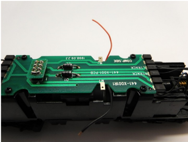
Platine plaatsen Mount the PCB Plaats de printplaat
