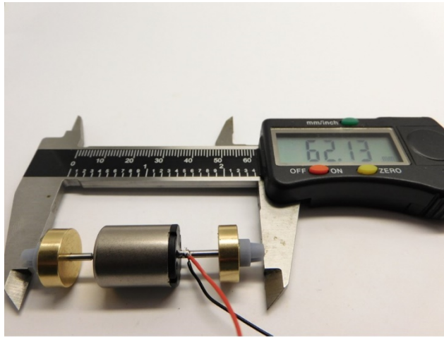
Kardankupplungshalter platzieren Mount cardan coupler pockets Plaats de cardan koppelings houders
