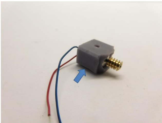
Die Ecken schräg feilen File the corners at an angle Vijl de hoeken schuin af
