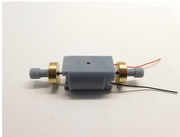
Kleben Sie die Kardankupplungen Glue the cardan couplings Verlijm de kardan koppelingen
