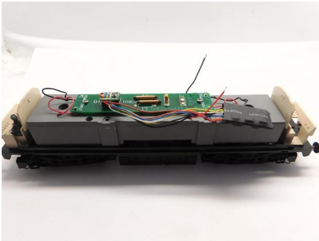
Platine platzieren Mount PCB Plaats de rintplaat
