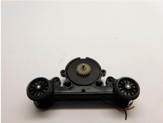
Motor platzieren Place the motor Motor plaatsen
