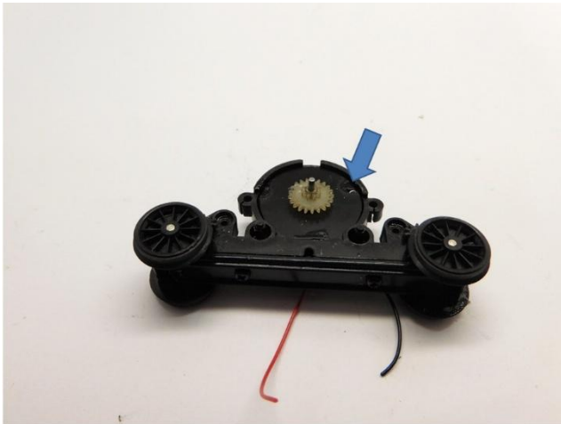
Der Motor wird mit Epoxidkleber oder Sekundenkleber geklebt The motor is glued with epoxy glue or super glue De motor wordt met epoxylijm of secondelijm verlijmd
